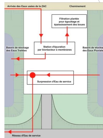
STATION D'EPURATION PAR BIOREACTEUR A MEMBRANES
